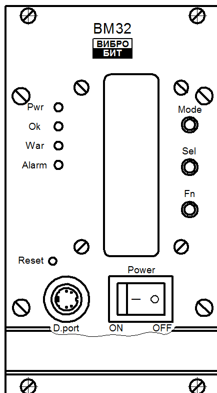
Рисунок 25 – Лицевая панель блока контроля ВМ32
