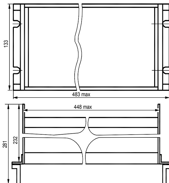
Рисунок В.4 – Каркас
