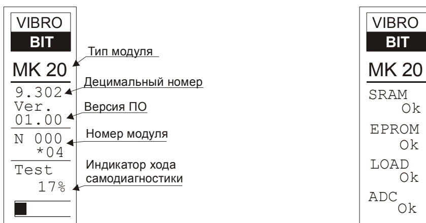
а) Стартовая информация на ЖКИ модуля МК20
