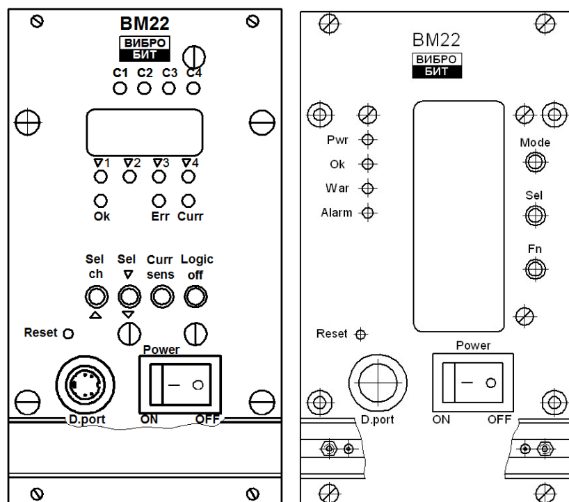
Рисунок Б.5 — Блоки контроля BM22
