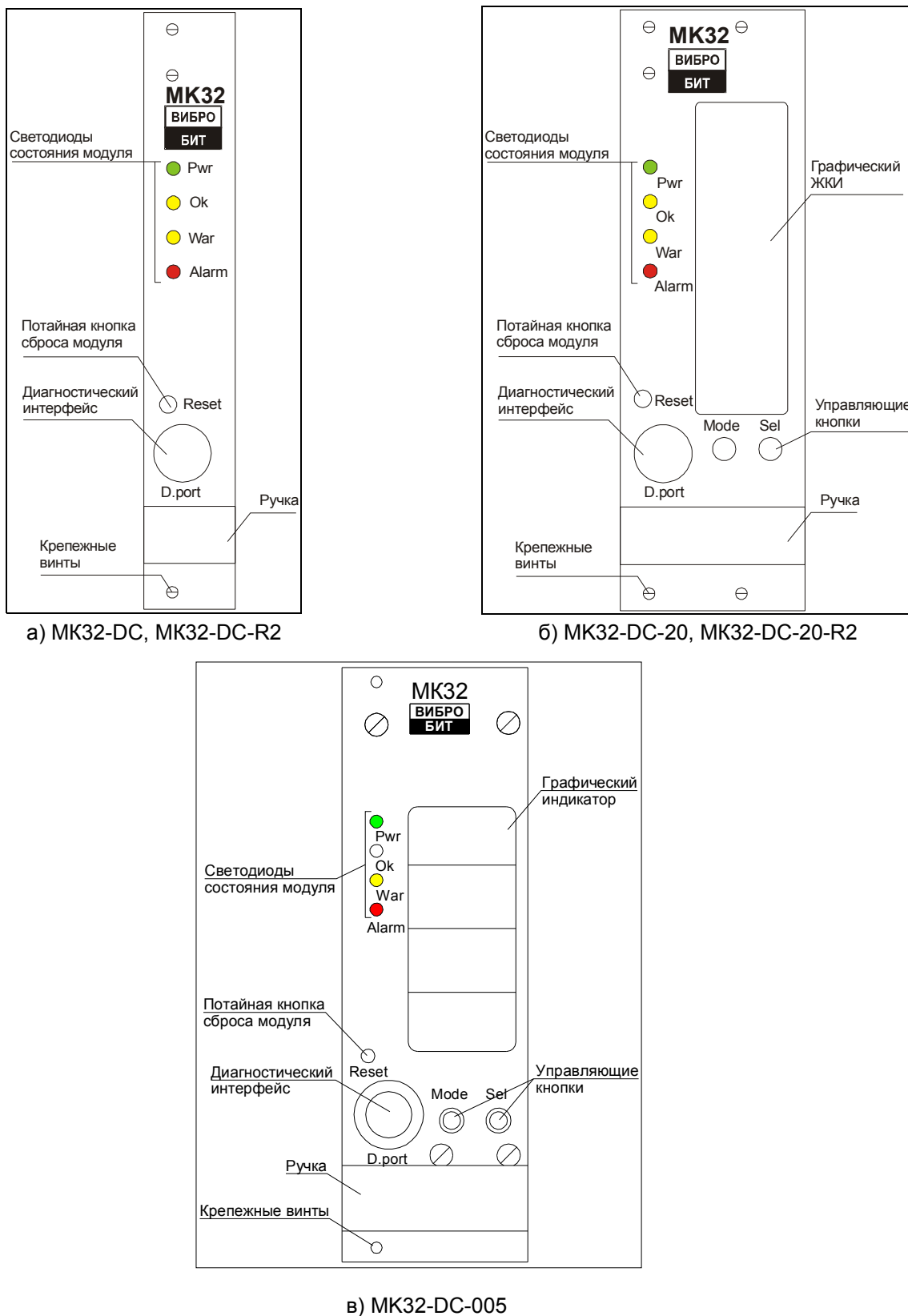
Рисунок 12 – Внешний вид лицевых панелей модуля МК32 в зависимости от кода маркировки
