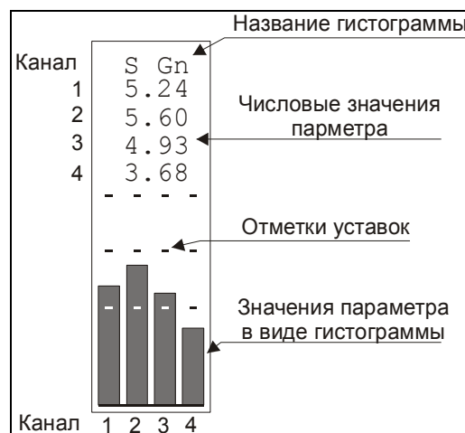
Рисунок 13 – Пример вывода данных в виде гистограммы для модуля МК32
