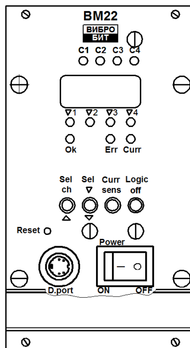
б) BM22 со светодиодным индикатором
