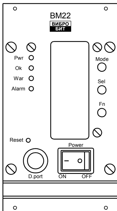
а) BM22 со специализированным ЖКИ
