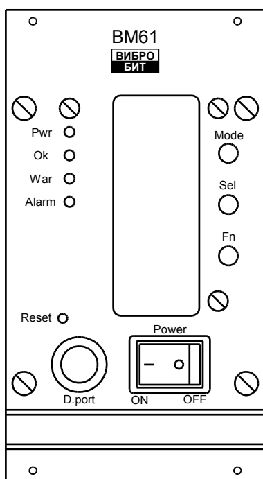
в) BM61 со специализированным ЖКИ
