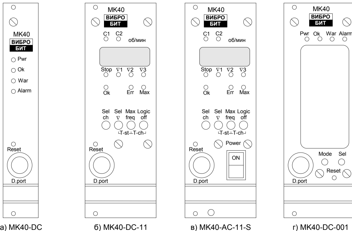
Рисунок 17 – Внешний вид лицевых панелей модуля МК40
