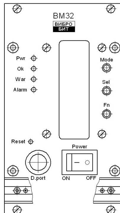
Рисунок Б.7 – Блок контроля BM32
