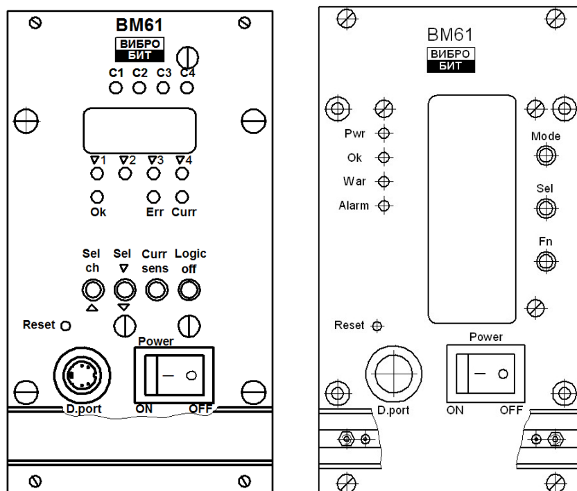
Рисунок Б.6 – Блоки контроля BM61
