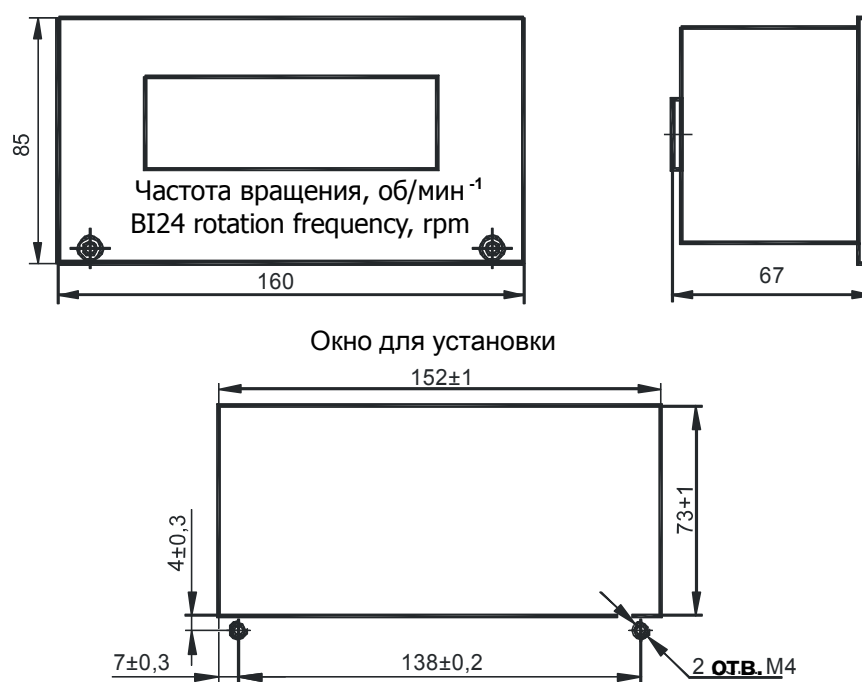
Рисунок В.2 – Блок индикации БИ24
