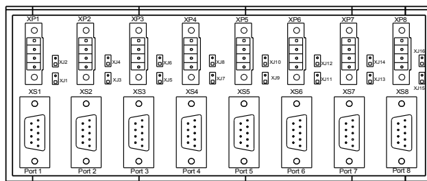
Рисунок 29 – Внешний вид блока коммутации DB9-MC-8
