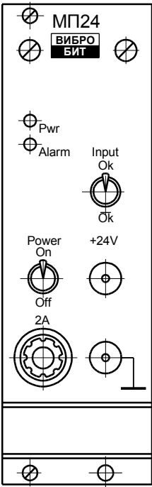
Рисунок Б.8 – Модуль питания МП24
