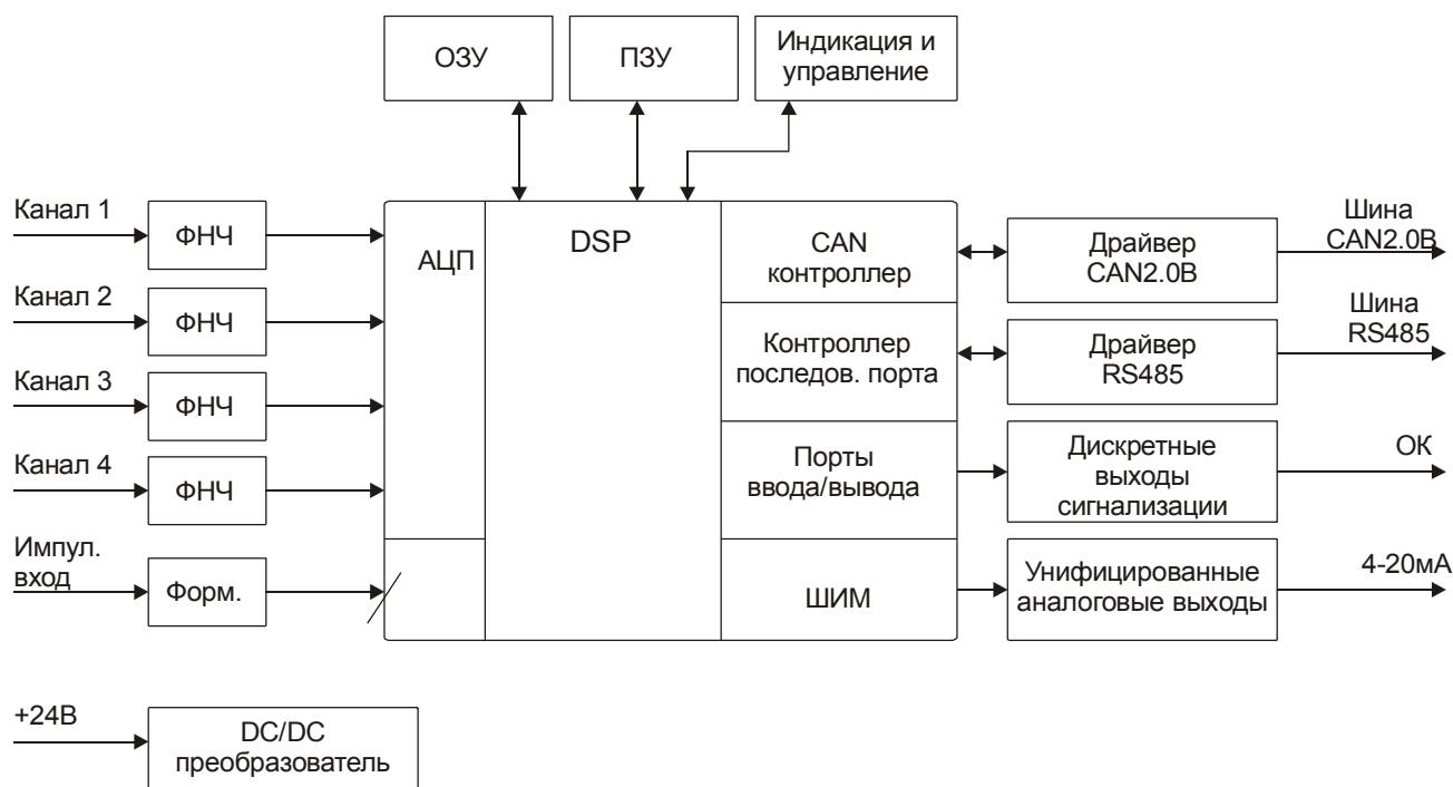
Рисунок 1 – Структурная схема модуля
