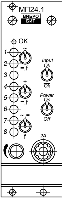
Рисунок Б.9 – Модуль питания МП24.1
