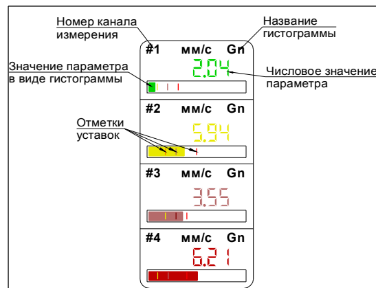
Рисунок 15 – Пример вывода данных в виде гистограммы для модуля МК32
