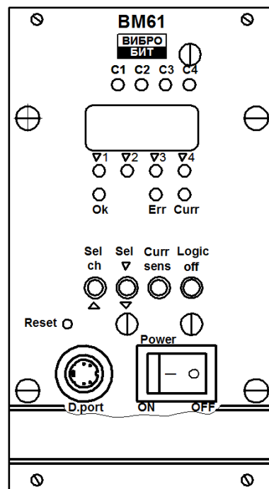
г) BM61 со светодиодным индикатором
