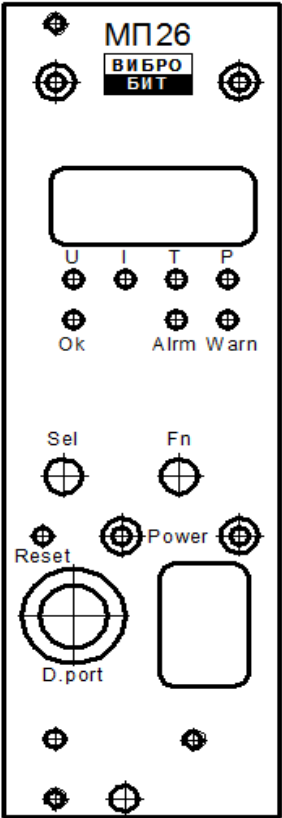
Рисунок Б.10 – Модуль питания МП26
