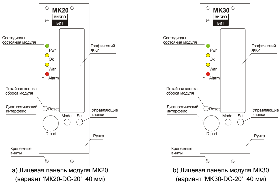
Рисунок 7 – Внешний вид лицевых панелей модулей МК20 и МК30
